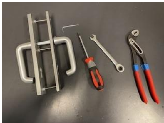
1.VHB AMI, benodigd gereedschap: kruiskop schroevendraaier, imbusleutel 5, waterpomptang of steeksleutel 10
