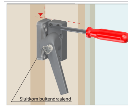
Tekening 4 bevestiging sluitkom
