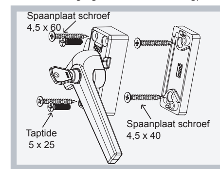
Tekening 5 gebruik zamac onderlegplaat
