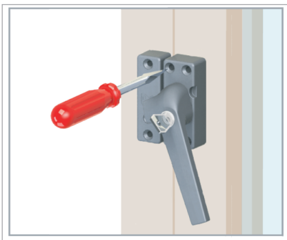
Tekening 2 Aftekenen bevestiging
