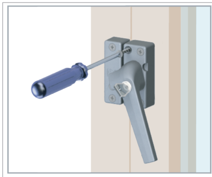
Tekening 3 Montage sluitkom
