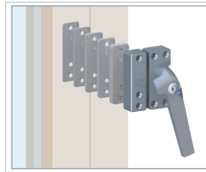
Tekening 4 Gebruik vulplaatjes (optie)
